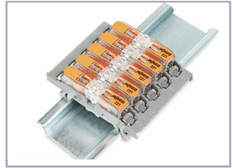
Befestigungsadapter ohne Zugentlastung, auf die Tragschiene aufgerastet
