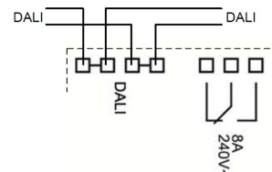
Anschlussplan RM16
