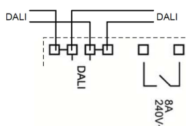
Anschlussplan RM8
