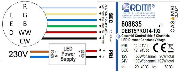
Typisches Schaltbild Typical connection scheme
