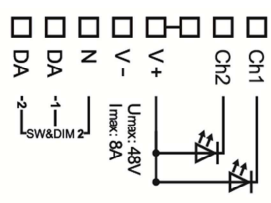
Anschlussplan Dose 8A
