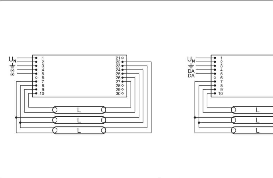
Verdrahtungsplan
