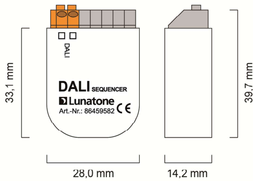
Abmessungen Dose
