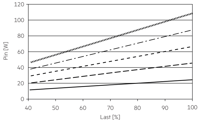
4.5.3 Eingangsleistung in Abhängigkeit zur Last 277 V, 60 Hz
