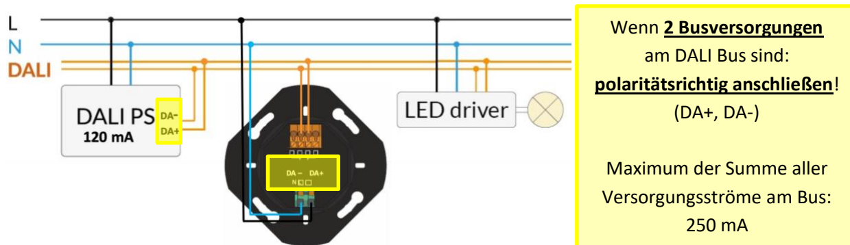
Abbildung 1 DALI-2 ROT PS – Beispielinstallation mit zweiter DALI PS am DALI Bus
