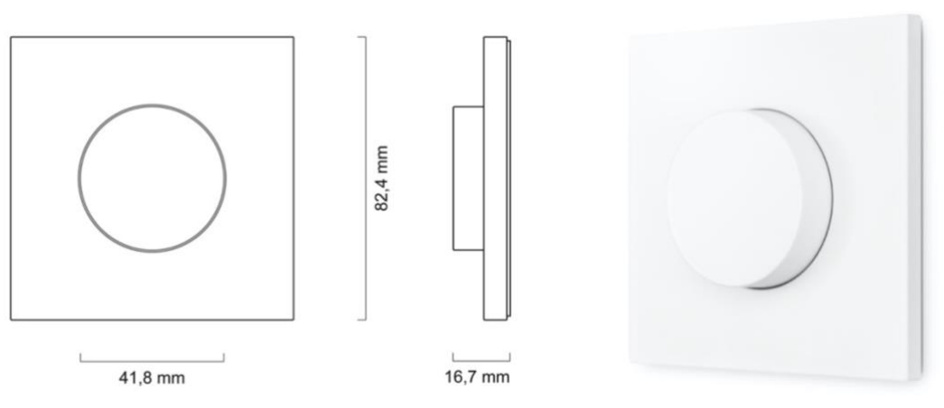
Abmessungen Drehschalter Abdeckung Lunatone (-Z04 & -Z05)
