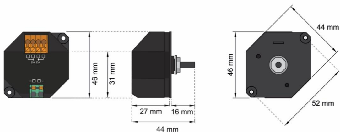
Abmessungen DALI-2 ROT PS CH: 86459822-D2-CH-PS
