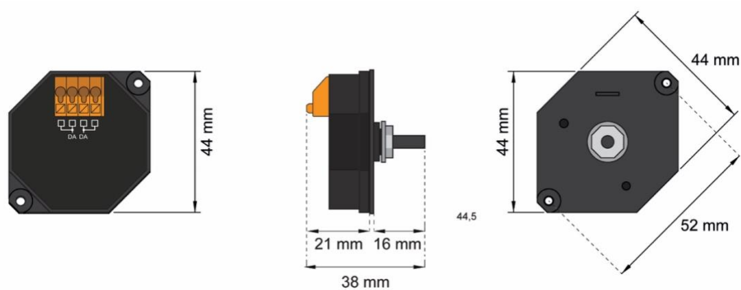
Abmessungen DALI-2 ROT CH: 86459822-D2-CH
