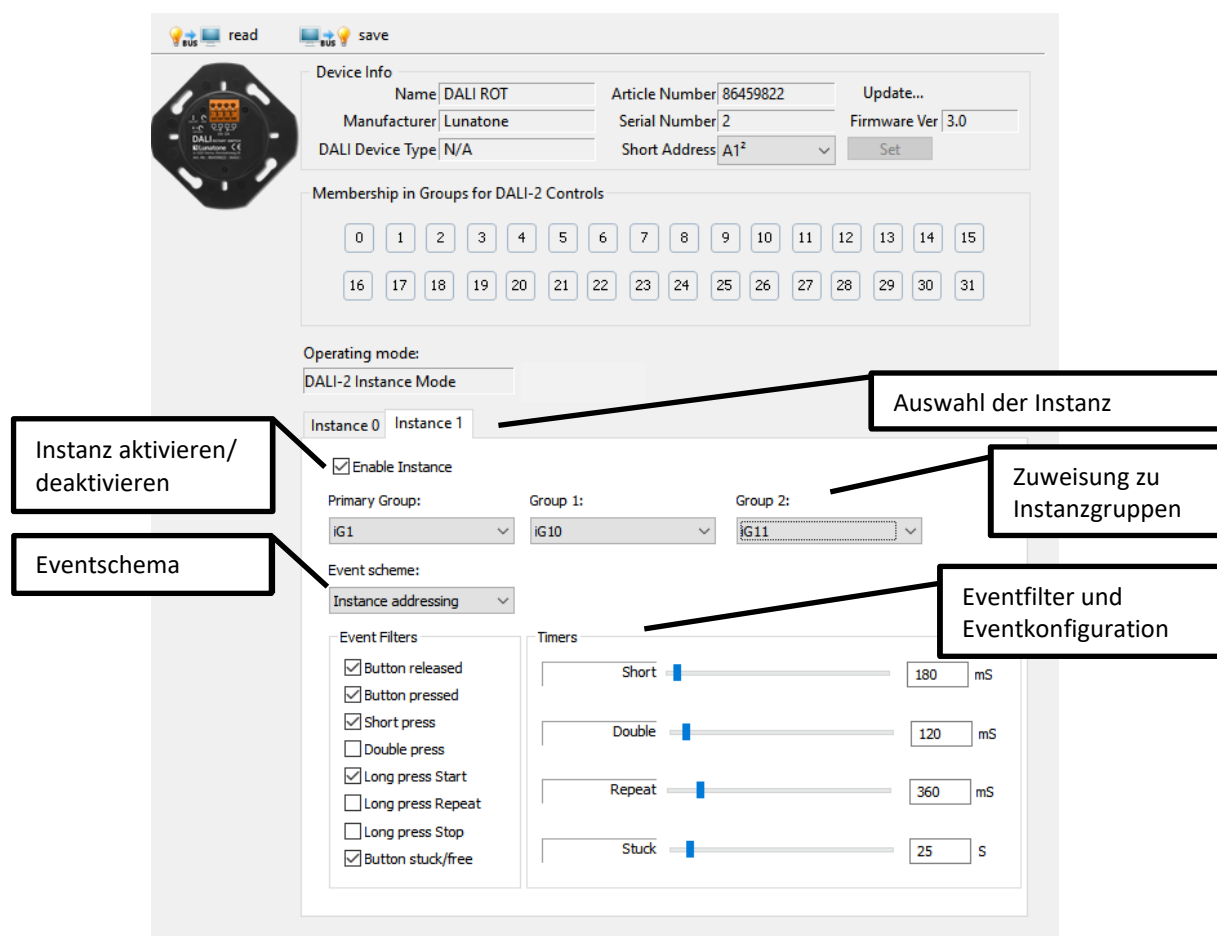
Abbildung 3 Einstell- und Konfigurationsmöglichkeiten: Instanzen
