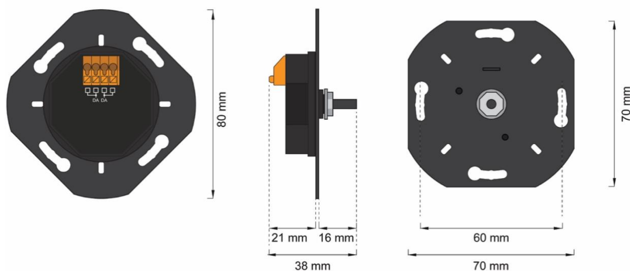
Abmessungen DALI-2 ROT: 86459822-D2
