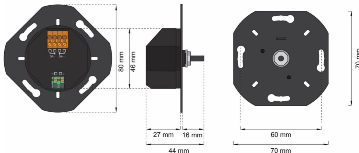
Abmessungen DALI-2 ROT PS: 86459822-D2-PS
