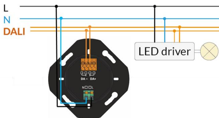
Beispielinstallation DALI-2 ROT PS
