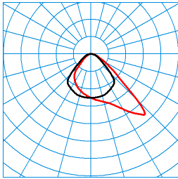
Bicult Act T G2 SMC TGCS 55 ETDI 03 EU (ACTCCW) TX369222 ■ C0 - C180 ■ C90 - C270 DIN 5040: D54 UTE: 0,10 D + 0,90 T CEN Flux Code: 59 89 98 10 100 82 96 100 90
