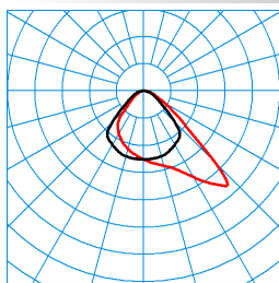
Bicult Act T G2 SMC TGCS 55 ETDI 03 EU (ACTCWW) TX369222 ■ C0 - C180 ■ C90 - C270 DIN 5040: D54 UTE: 0,10 D + 0,90 T CEN Flux Code: 59 89 98 10 100 82 96 100 90
