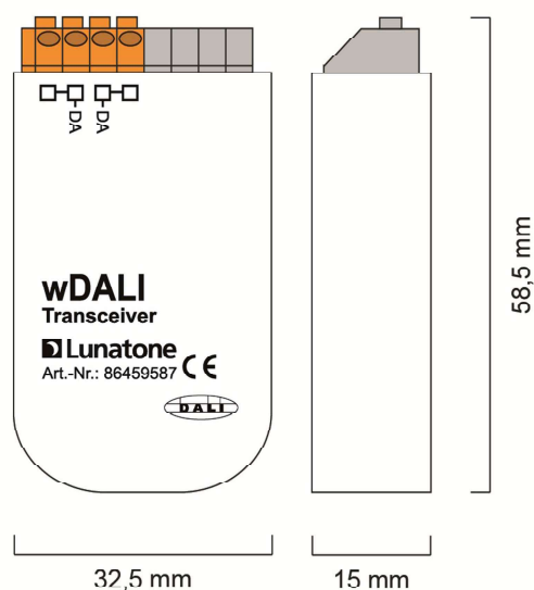
Geometrie Transceiver (Empfangseingheit)
