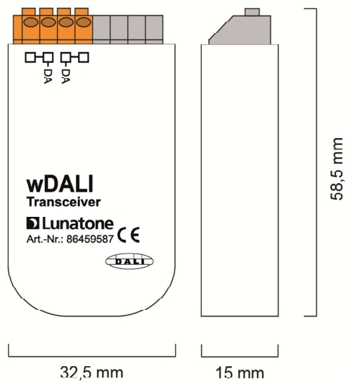
Geometrie Transceiver (Empfangseinheit)
