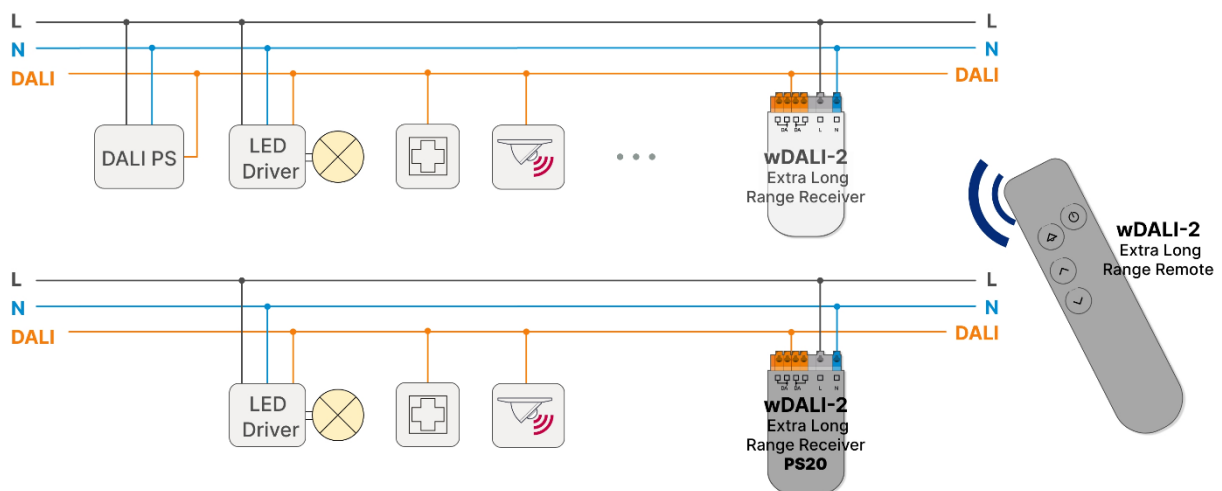
Abb. 1 typische Anwendung: drahtlose Steuerung eines DALI Systems
