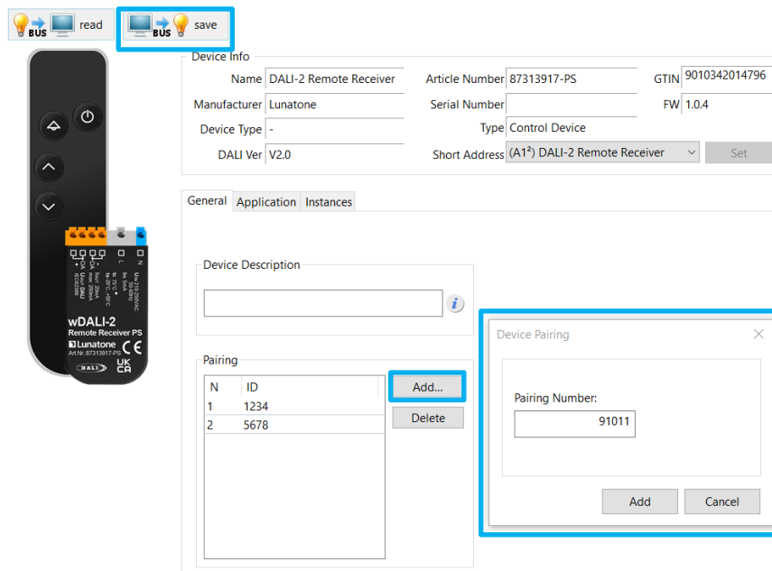
Abb. 2.: Koppeln von Remote und Receiver
