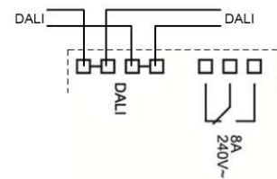
Anschlussplan RM16
