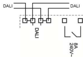
Anschlussplan RM8
