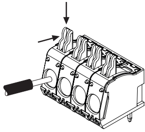
Eingangsklemmen
