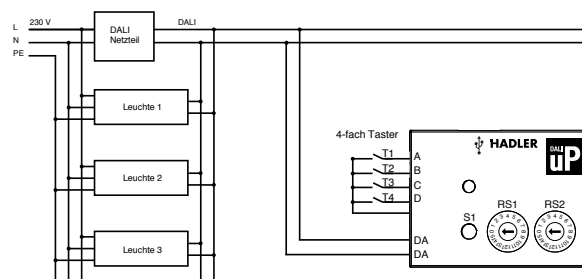
DALI uP Verdrahtungsplan
