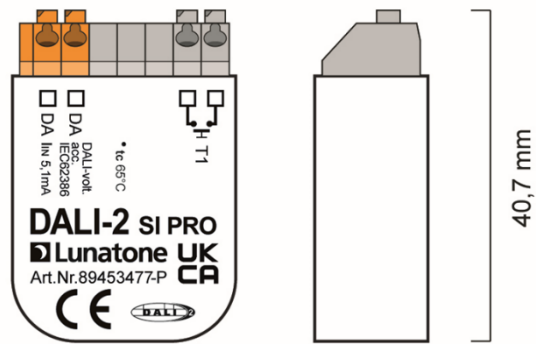
28 mm 14,2 mm dimensions DALI-2 SI PRO
