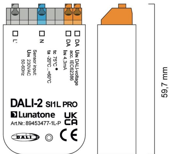
32,8 mm 15,2 mm dimensions DALI-2 SI 1L PRO
