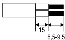
H03VH2-F 0,75 mm 2
