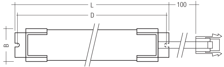
Bild 1: Stab
