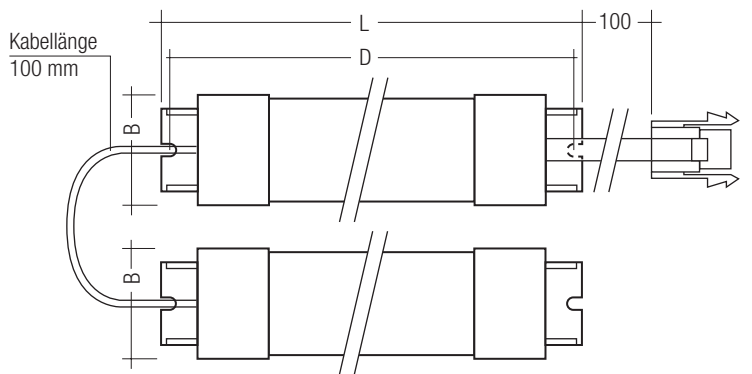
Bild 2: Stab + Stab
