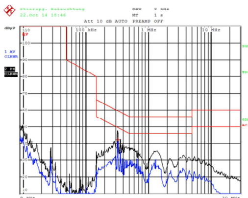
Messung Netzleitung
