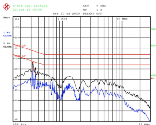
Messung DALI Leitung
