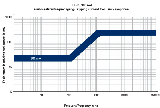
Diagramme Fehlerstromschutzschalter DFS 4 080-4/0,30-B SK R
