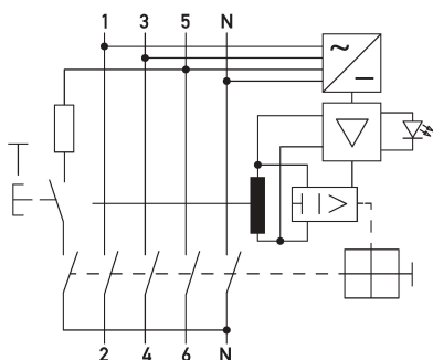
Schaltungsbeispiel Fehlerstromschutzschalter DFS 4 080-4/0,30-B SK R
