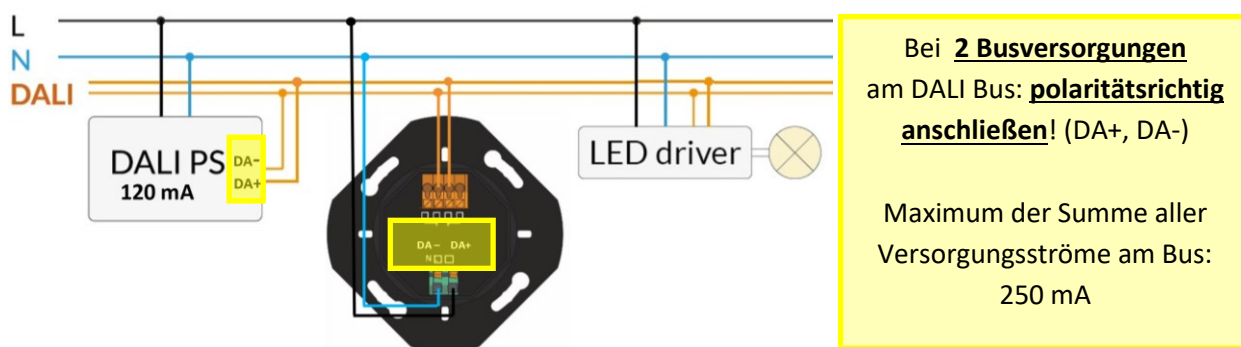
Abb. 1 DALI-2 ROT PS – Beispielinstallation mit zweiter DALI PS am DALI Bus
