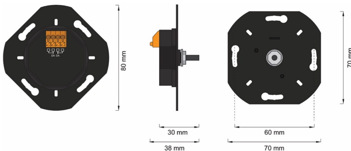
Abmessungen Drehschalter
