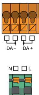
Anschlussplan DALI-2 ROT Touch PS
