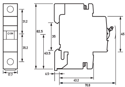
Maßzeichnung Leitungsschutzschalter DLS 6hdc C63-1
