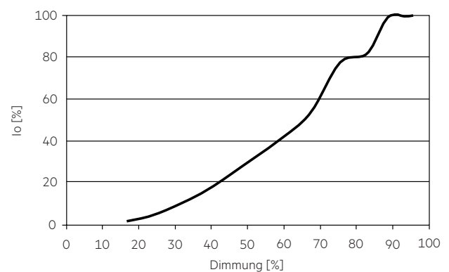
4.1.6 Phase-cut Dimmungskurve (benötigt Dimmer)
